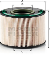
Fuel Filter PU 1040 x EM-20048
