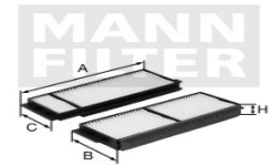
Cabin Air Filter CU 2011-2 EM-40209
